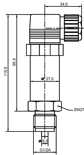
P 10 G 1/2A DIN 16288
