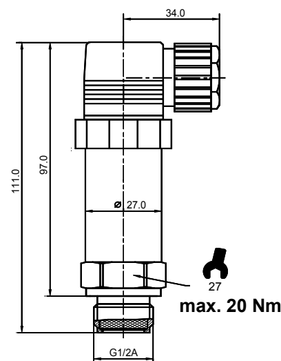
P 20 G 1/2A DIN 3852
