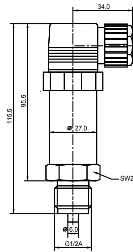
P 10 G 1/2A DIN 16288
