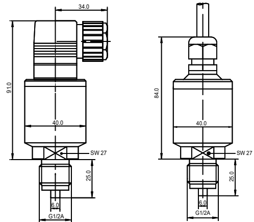
P 121 G 1/2A DIN 16288
